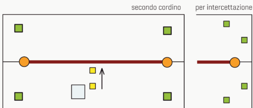
Linea vita unidirezionale a singola campata
