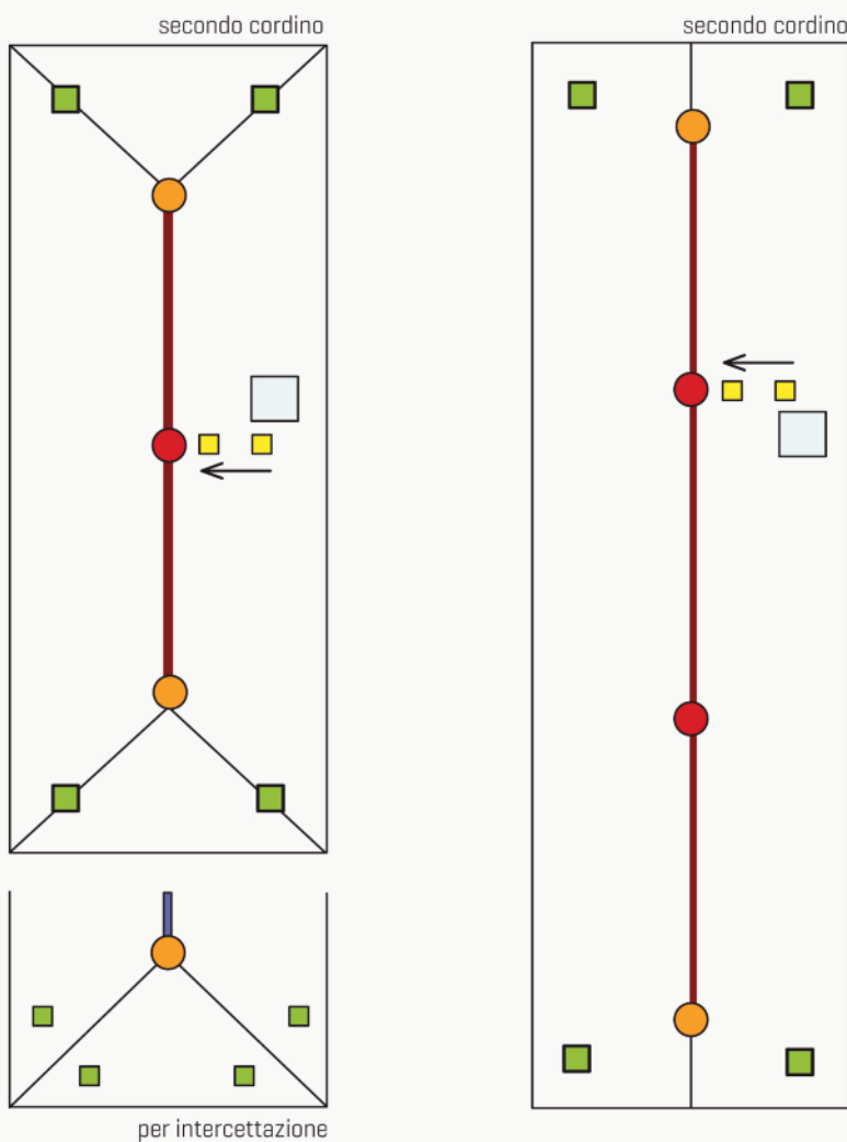
Linea vita unidirezionale a più campate
