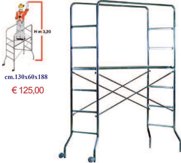
Mini ponteggio zincato TRIO . Altezza massima con operatore Mt. 3,20.
