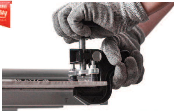
Pinza troncatrice alti spessori "169TBRAI", utilizzata in abbinamento alle taglierine grandi formati. Blister appendibile.
